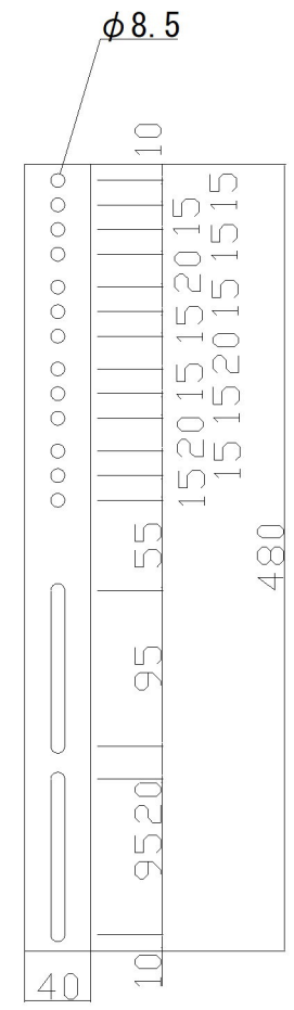
アタッチメント穴位置図
