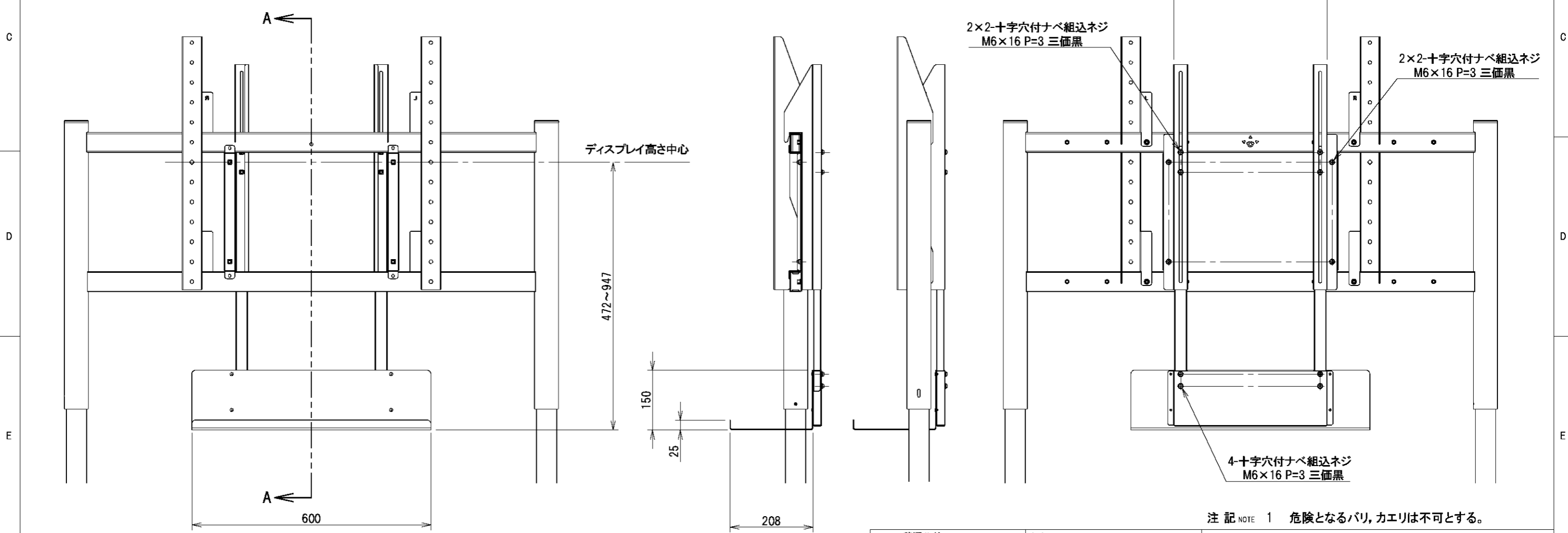
断面図 A-A
