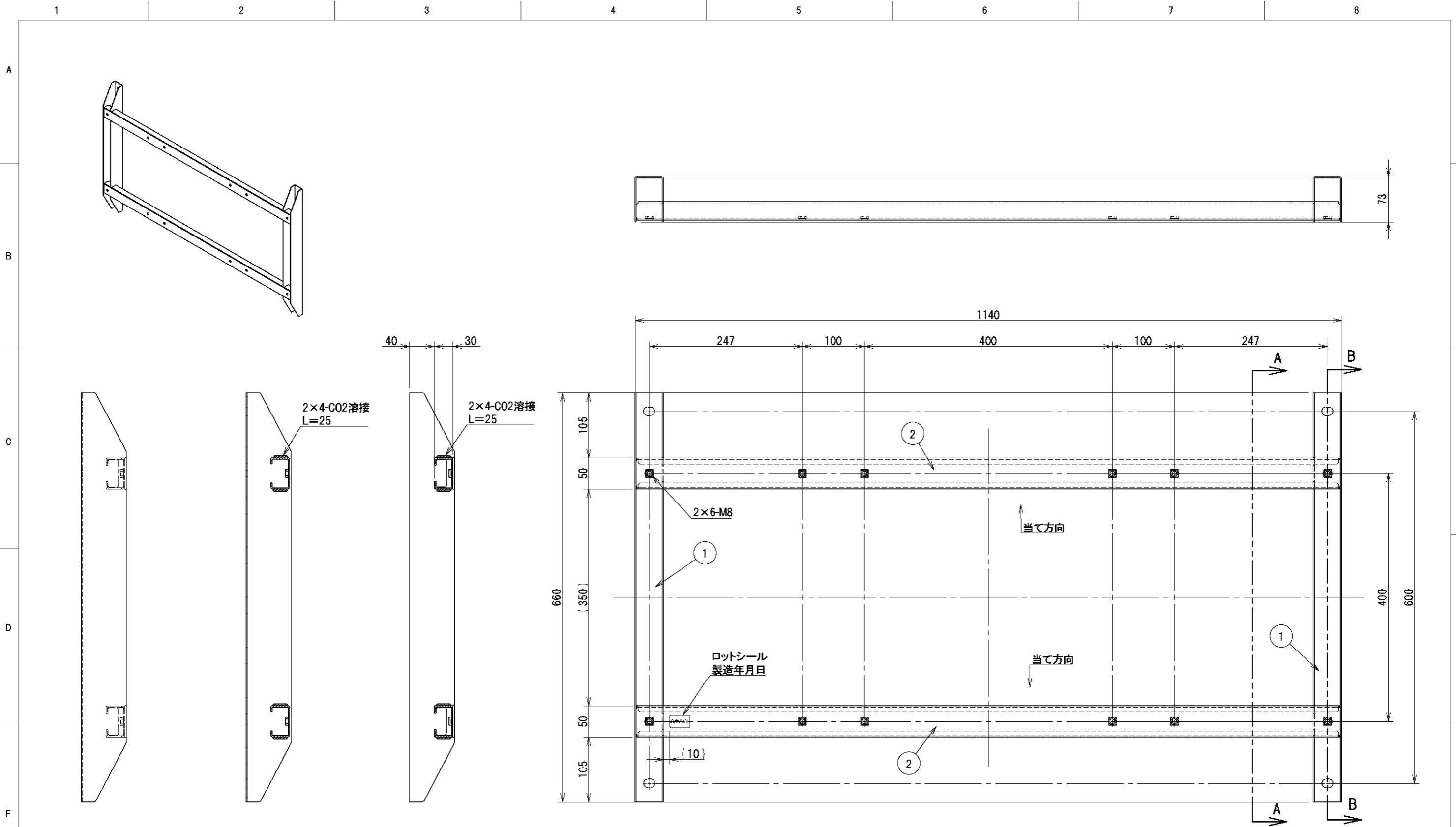
B-B断面図(S:1/6)
