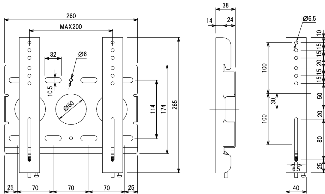
アタッチメント穴位置図
