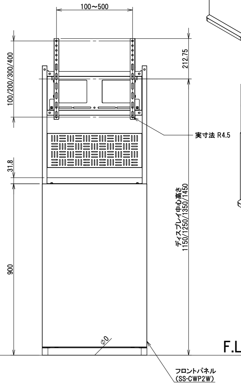
断面図 A-A
