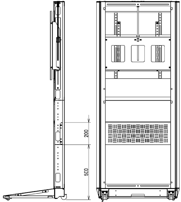
断面図 A-A
